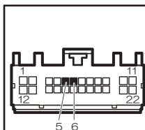
オーディオユニット 22P コネクター
