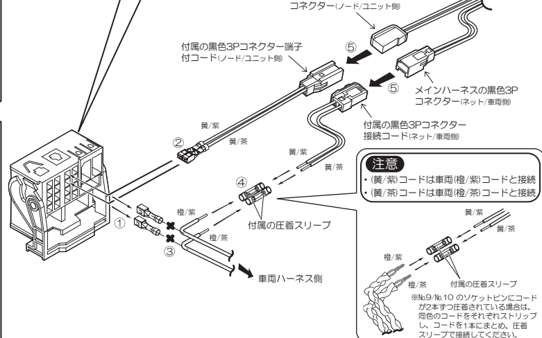
図2 (ハーネス側)
