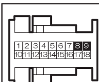
ナビゲーション ディスプレイユニット 黒色 18P コネクター
