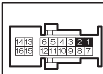
エアコン コントロールユニット 16P コネクター
