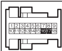
エアコン コントロールユニット 18P コネクター
