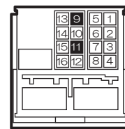
オーディオユニット 40P コネクター
