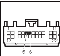
オーディオユニット 22P コネクター
