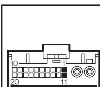
オーディオユニット裏 20P コネクター
